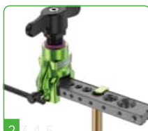
2 Rura miedziana wchodzi do otworu, a płytka ograniczająca znajduje się na rurze miedzianej
